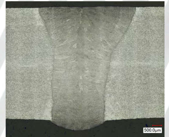
Сварочный шов в поперечном сечении – минимальное тепловложение и максимальное качество сварки
